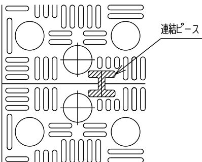
連結図
